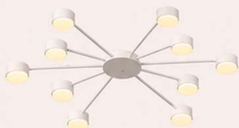
XG1254-10 840 × 740 × 70 mm 10 × GX53 · 15W
